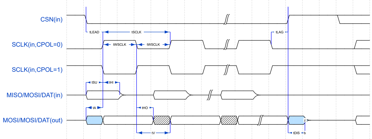
图 25: SPI 从模式时序 (CPHA=0)
